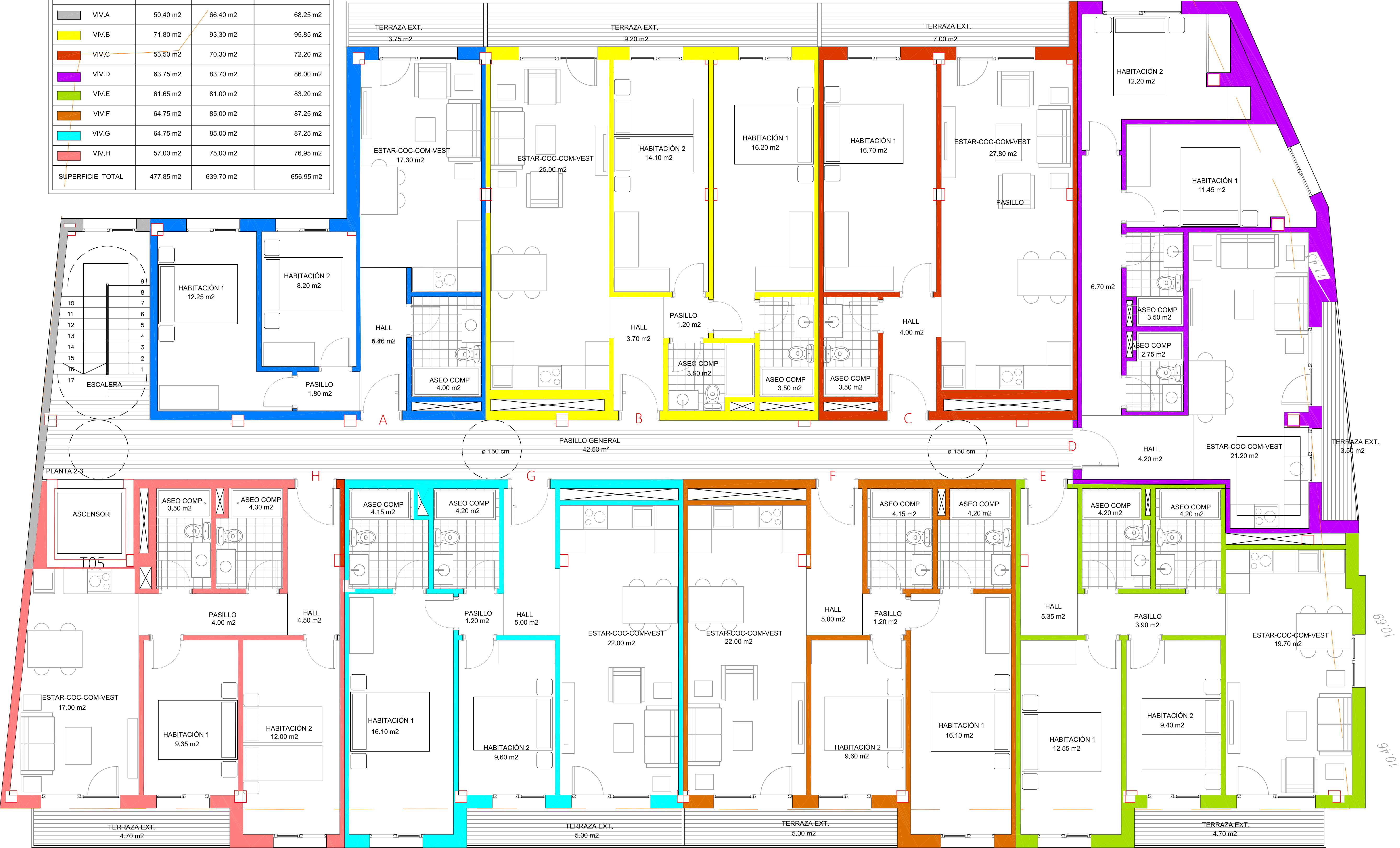
PLANTA 2-3
