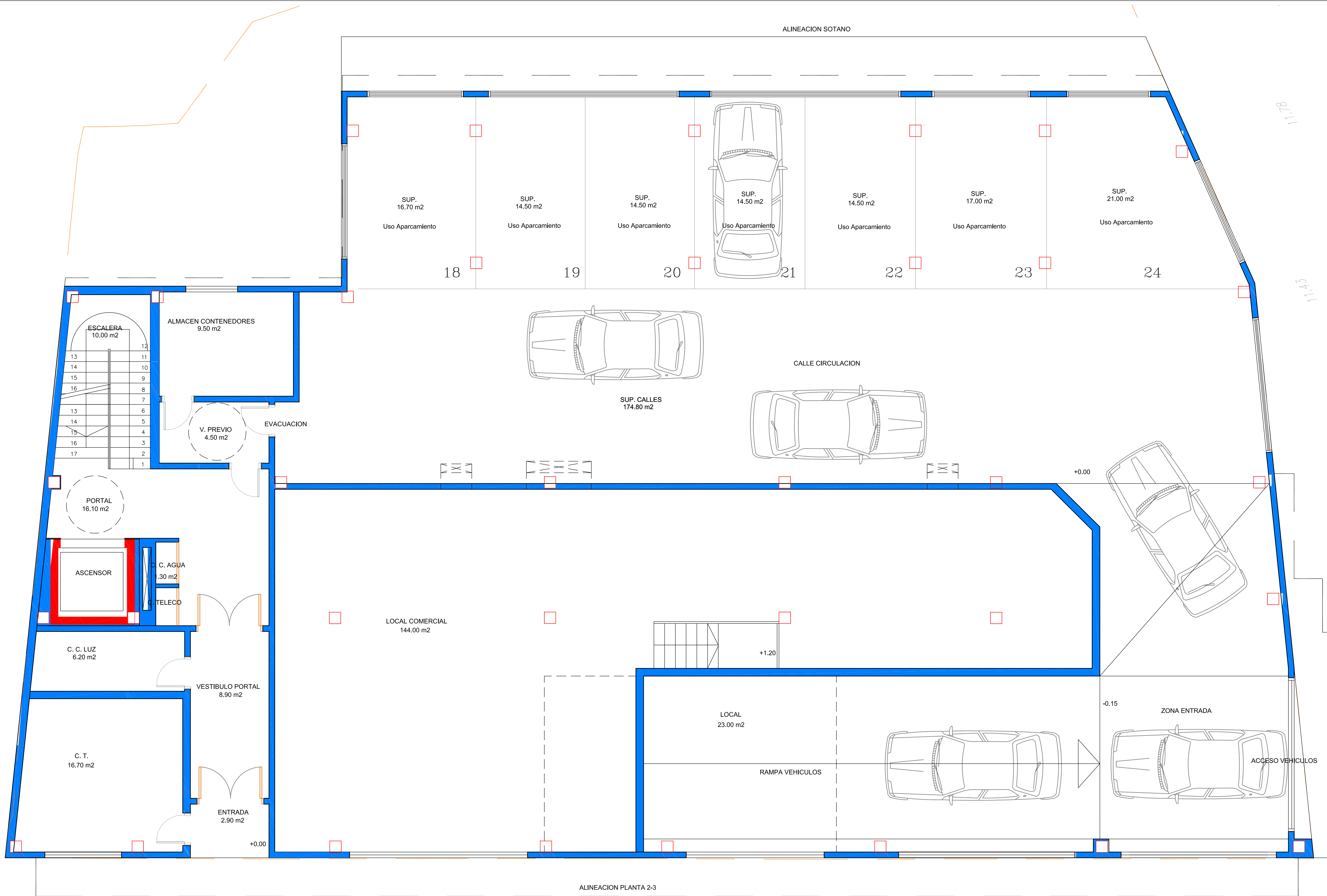
PLANTA BAJA SUP. CONST. 603,00 m 2
